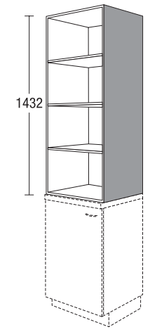
Aufsatzregal Höhe: 1432 mm Breite: 600, 650 mm
