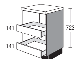
Unterschrank für Getränkekekisten Höhe: 723 mm Breite: 600 mm
