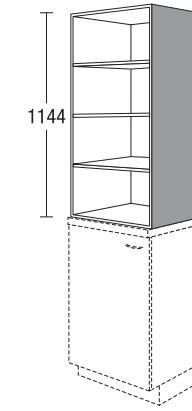
Aufsatzregal Höhe: 1144 mm Breite: 600, 650 mm
