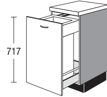
Unterschrank mit Wertstoffsammler Höhe: 723 mm Breite: 400 mm
